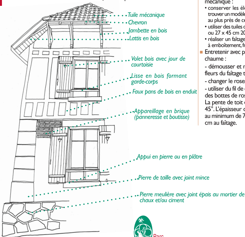
Exemple d'une façade composite
