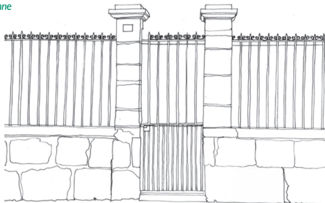
Piles maçonnées pour intégration du portail
